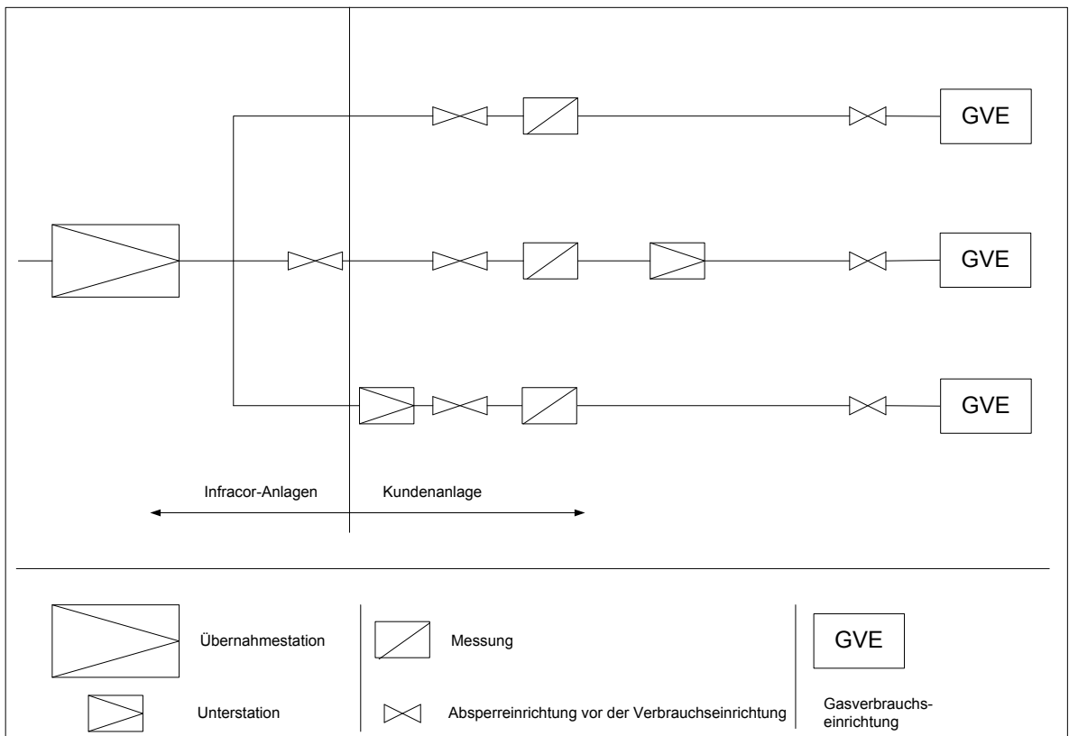
Bild 5: Schnittstellen EvD-Anlagen / Kundenanlagen
