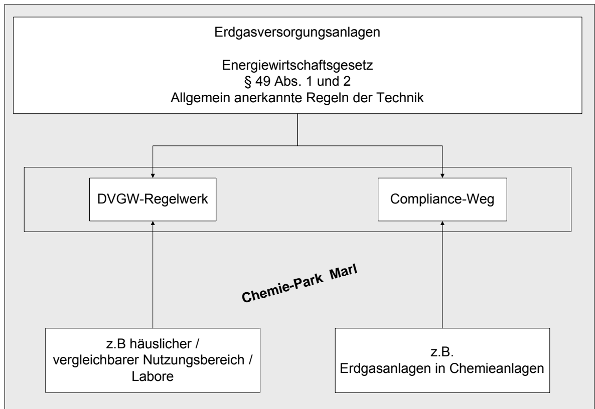
Bild 1: Anwendung DVGW-Regelwerk und Compliance-Weg
