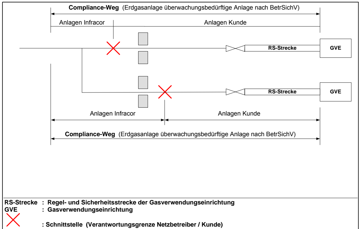
Bild 2: Compliance-Weg, z.B. für eine Erdgasversorgungseinrichtung in einer Chemieanlage
