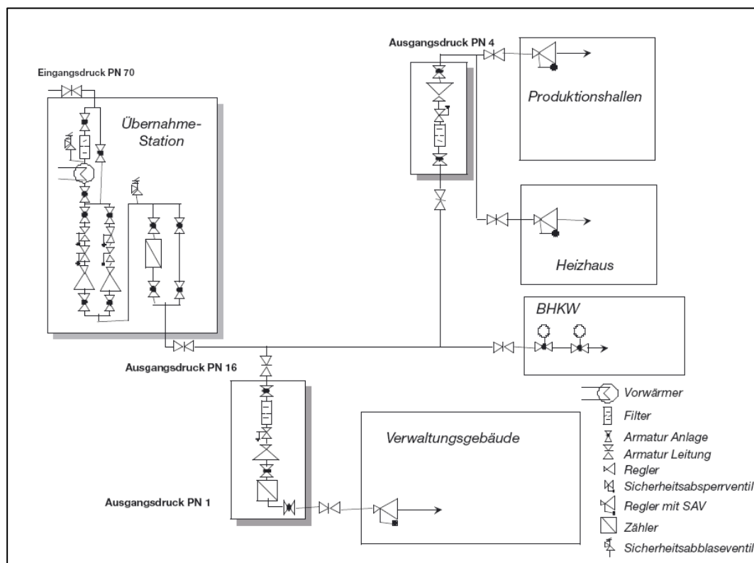
Bild 4: Aufbau der Gasversorgungsanlagen im Chemiepark Marl.
