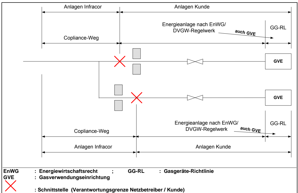
Bild 3: DVGW-Weg, z.B. häusliche/vergleichbare Anwendung
